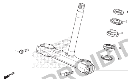
C-9 Coluna de Direção
