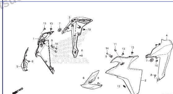
C-22 Carenagem
