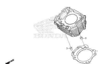
M-5 Cilindro
