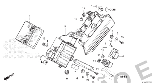
C-39.30 Tubo Lateral Dianteiro
