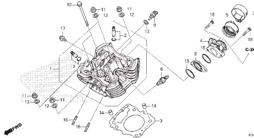
M-5 Cilindro
