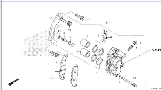
C-12 Cáliper do Freio Dianteiro
