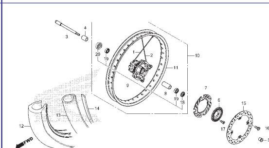
C-14.20 Roda Dianteira
