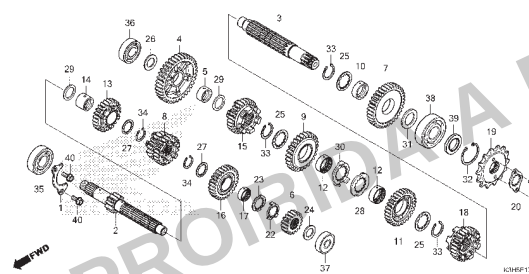
M-17 Transmissão
