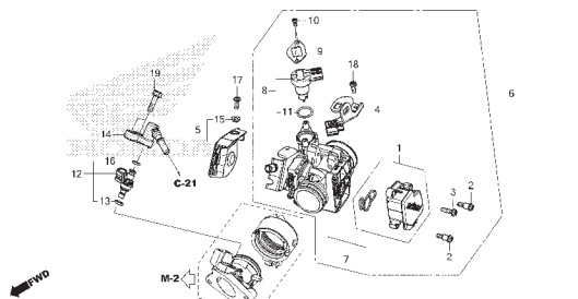
M-23 Corpo do Acelerador • Injetor
